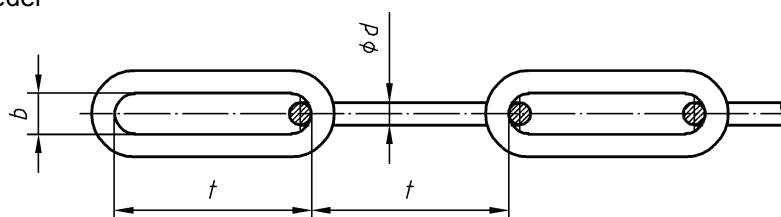
Bild 1 — Kette mit geraden Gliedern
