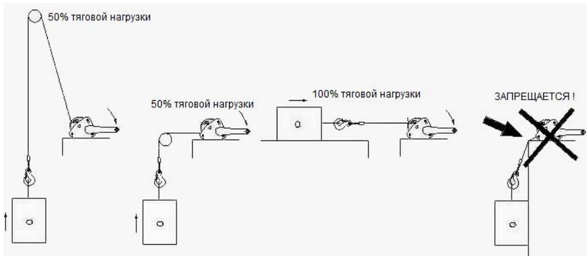
Рис. 3 - Использование блоков
